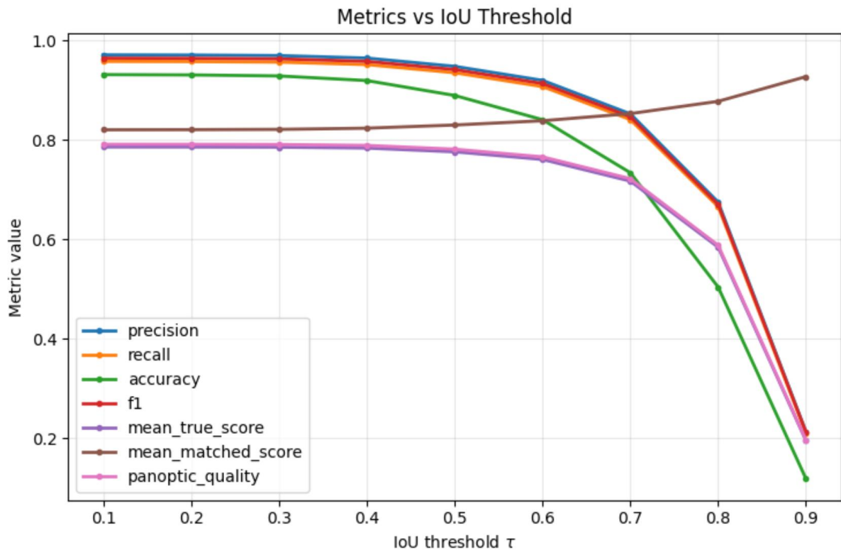
Hình 3.1 Sự biến thiên các chỉ số đánh giá của StarDist theo ngưỡng IoU.
